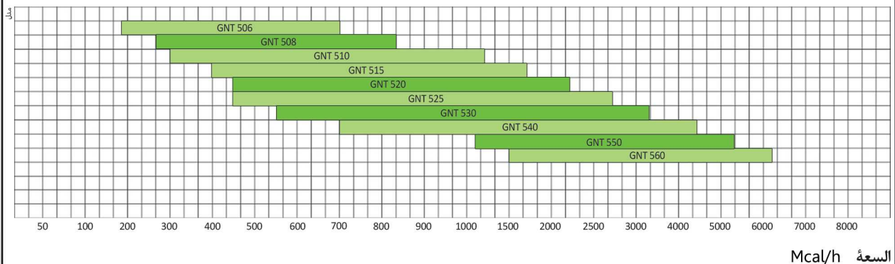
مشاعل ثلاثية الوقود (غاز - ديزل - مازوت)
