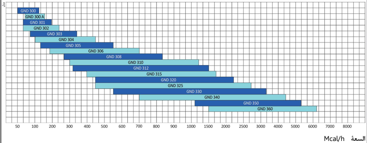
مشاعل ثنائية الوقود (غاز - ديزل)
