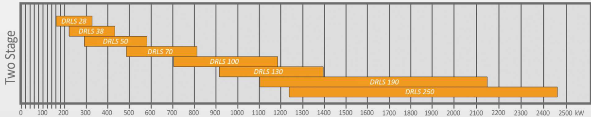
مخطط اختيار سعة مشاعل ريلو
