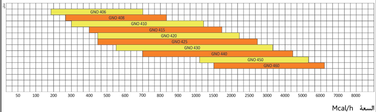
مشاعل تعمل بالمازوت
